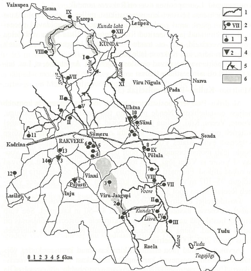
Joonis 2. Karst ja allikad: 1 – jõgi; 2 – mõõtmisprofiil; 3 – allikas; 4 – karst; 5 – pum-pamispunkt; 6 – kaitseala.
